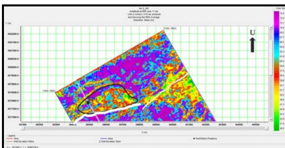
Gambar 19. Slice Map hasil inversi \mu -rho
