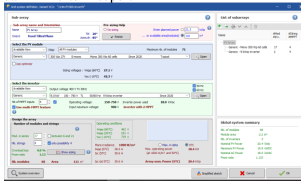
Gambar 4. Parameter Sistem
