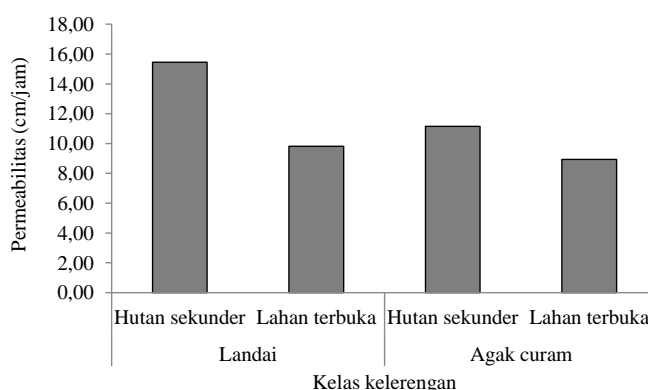
Gambar 5. Permeabilitas Tanah pada Kelas Kelerengannya Berbeda.
