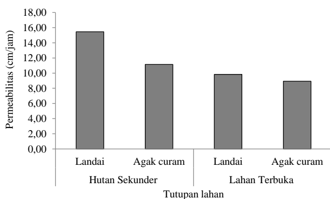
Gambar 4. Permeabilitas Tanah pada Tutupan Lahan Berbeda.
