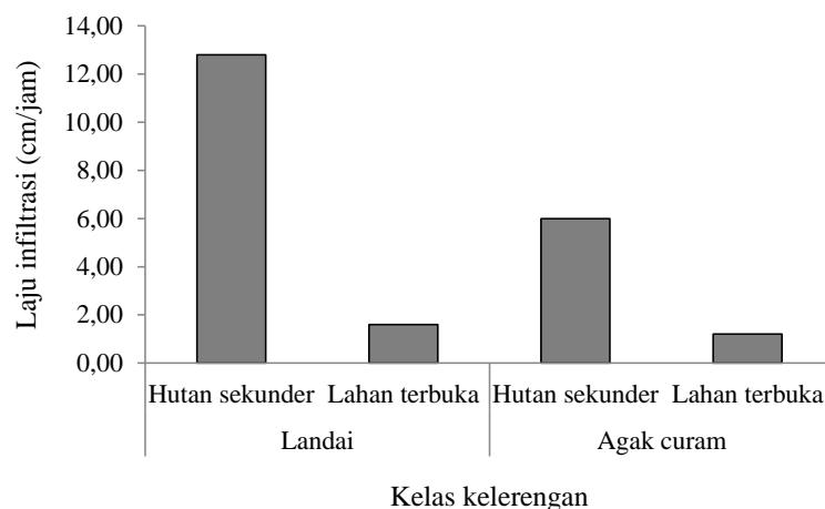
Gambar 3. Laju Infiltrasi pada Kelas Kelerengan Berbeda
