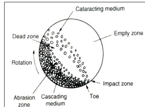
Gambar 3. Pergerakan material dalam Ball Mill
