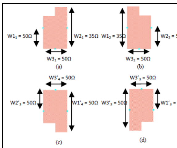
Gambar 2. Geometri dari T-junction yang digunakan. (a). T-junction dengan W1_1 = 50\Omega , W2_1 = 35\Omega , W3_1 = 50\Omega . (b). T-junction dengan W1_2 = 35\Omega , W2_2 = 50\Omega ,
