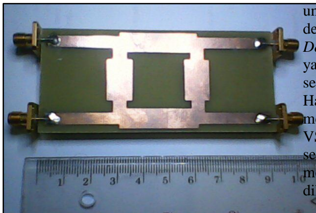
Gambar 10. Rangkaian Coupler
