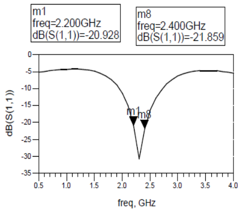
Gambar 6. Simulasi return loss untuk bandwidth
