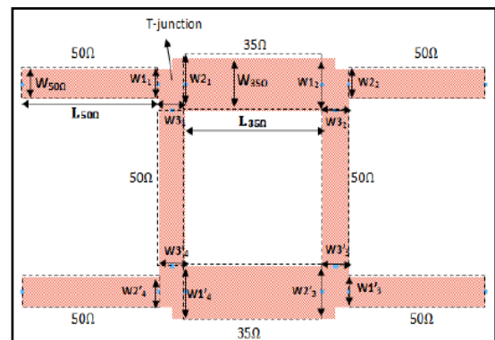
Gambar 3. Rangkaian microstrip branch line coupler dengan T-junction
