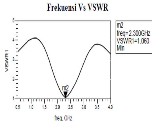
Gambar 5. Hasil simulasi VSWR
