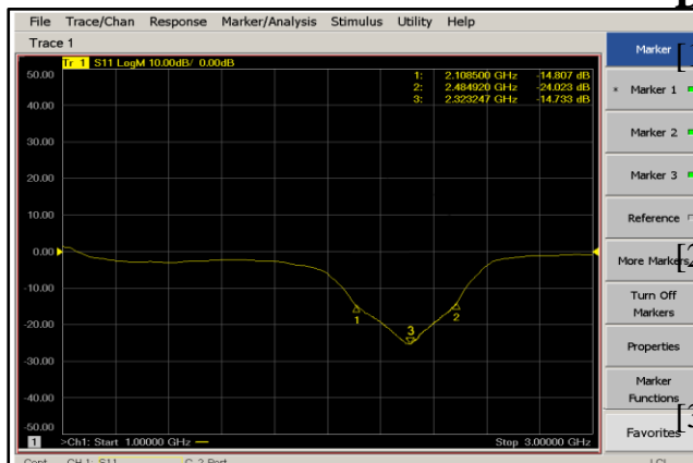
Gambar 11. Hasil Pengukuran Coupler
