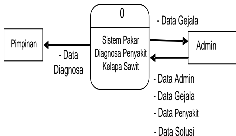
Gambar 2. Diagram Konteks
