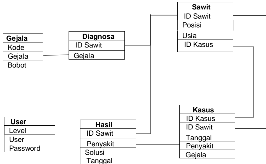
Gambar 4. Tabel dan Relasi
