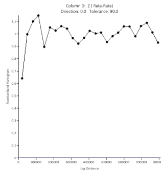
Gambar 1. Plotting Data Curah Hujan
