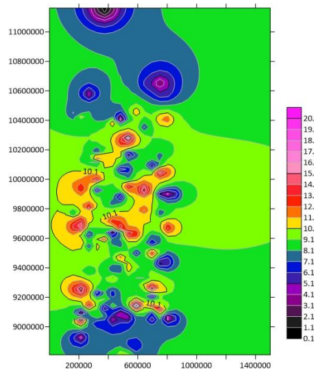
Gambar 3. Peta Kontur Data curah hujan bulanan
