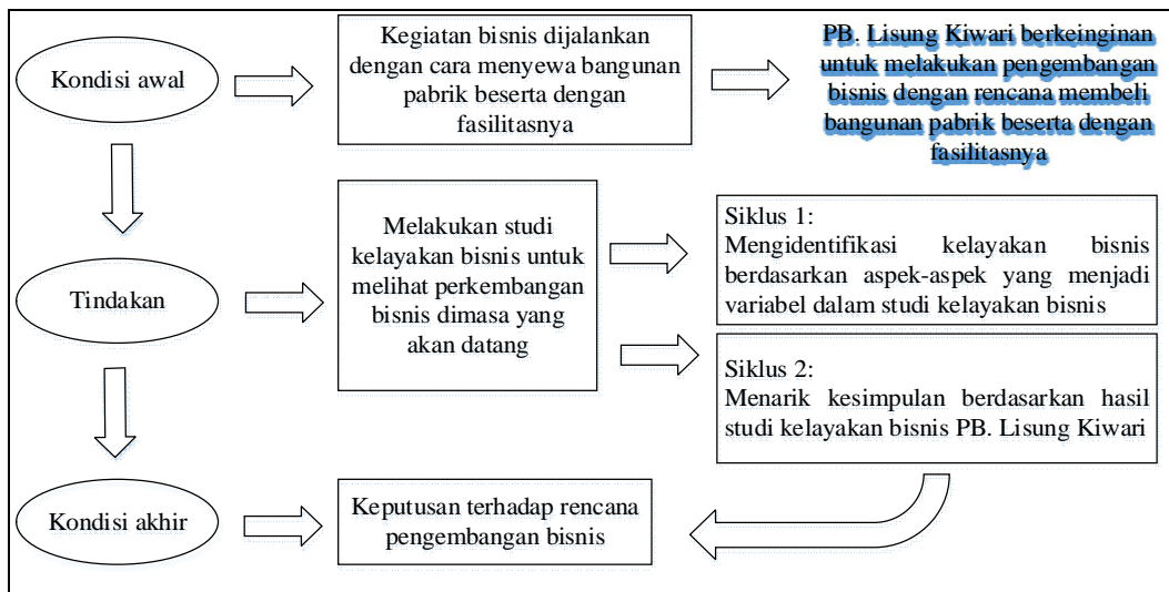
Gambar 2. Metodologi Penelitian
