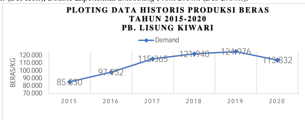
Gambar 3. Pola data
