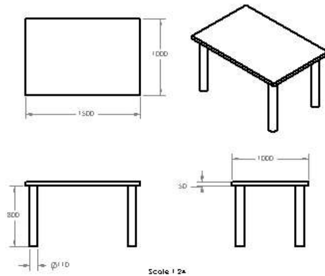
Gambar 4 Dimensi Meja Usulan Perbaikan Proses Pengepakan
