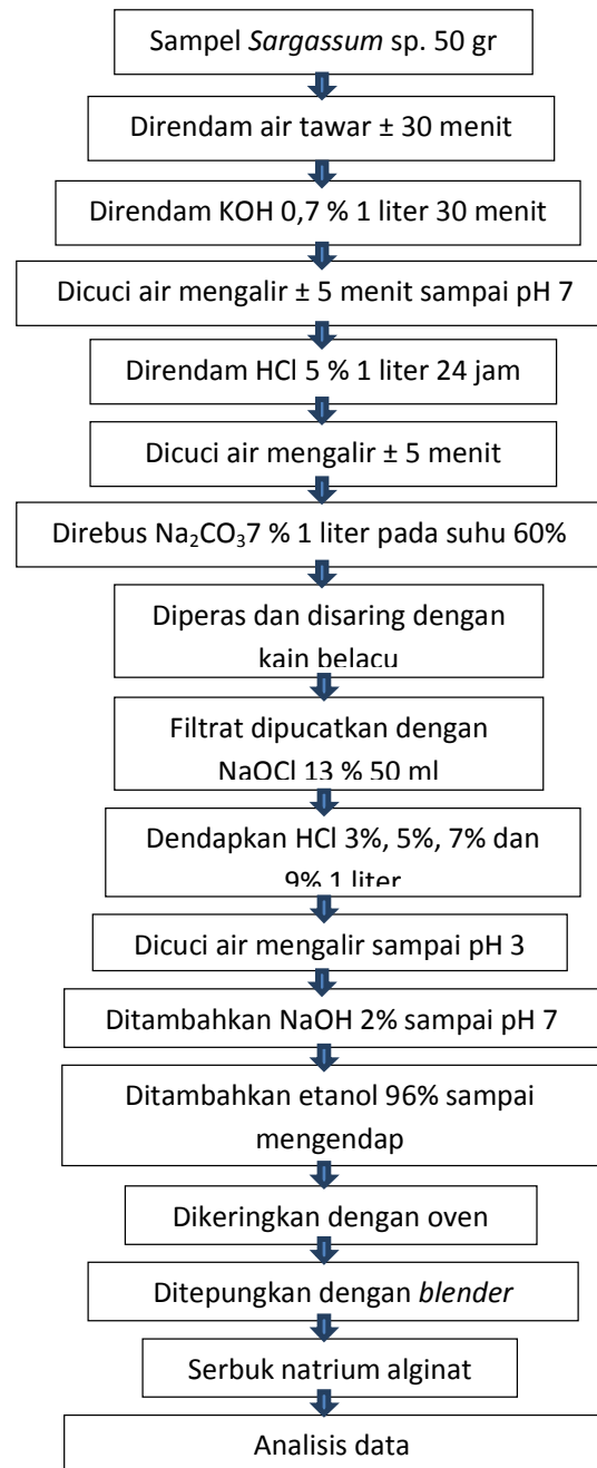
Gambar 2. Skema Alur Proses Ekstraksi Natrium Alginat Sargassum sp.
