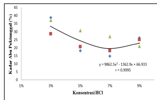
Gambar 10. Grafik Regresi Kadar Abu Natrium Alginat Rumput Laut Sargassum sp. dari Perairan Poktunggal pada Konsentrasi HCl yang Berbeda.
