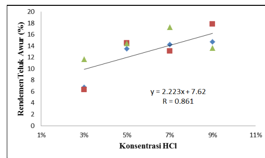
Gambar 3. Grafik Regresi Linier Rendemen Natrium Alginat Rumput Laut Sargassum sp. dari Perairan Teluk Awur pada Konsentrasi HCl yang Berbeda.
