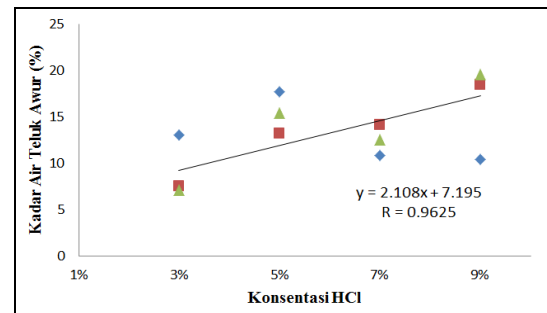
Gambar 7. Grafik Regresi Linier Kadar Air Natrium Alginat Rumput Laut Sargassum sp. dari Perairan Teluk Awur pada Konsentrasi HCl yang Berbeda.
