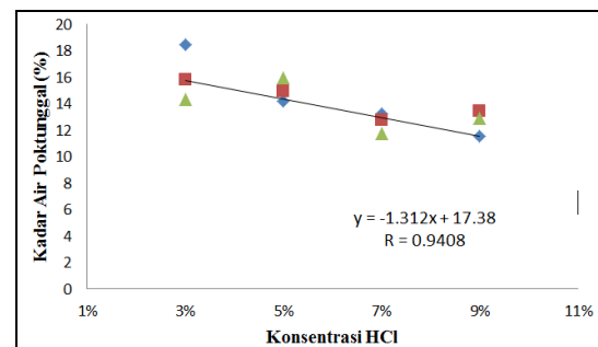
Gambar 8. Grafik Regresi Linier Kadar Air Natrium Alginat Rumput Laut Sargassum sp. dari Perairan Poktunggal pada Konsentrasi HCl yang Berbeda
