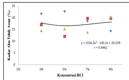
Gambar 9. Grafik Regresi Polinomial Kadar Abu Natrium Alginat Rumput Laut Sargassum sp. dari Perairan Teluk Awur pada Konsentrasi HCl yang Berbeda.
