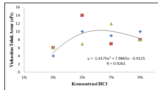
Gambar 5. Grafik Regresi Viskositas Natrium Alginat Rumput Laut Sargassum sp. dari Perairan Teluk Awur pada Konsentrasi HCl yang Berbeda.
