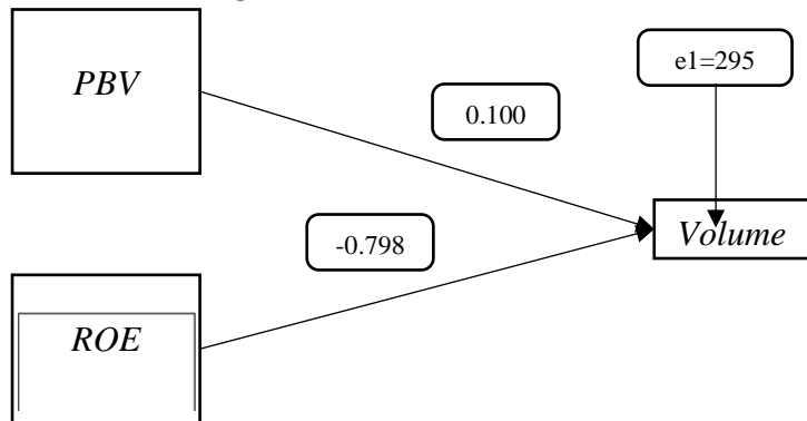
Gambar 2. Diagram Jalur Model Struktur I
