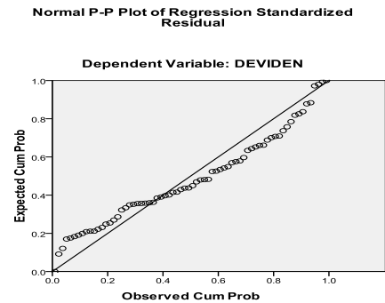
Gambar 1 Uji Normalitas
