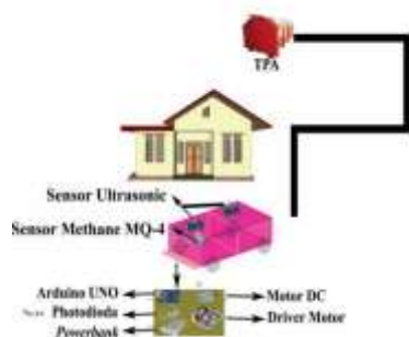
Gambar 7 Rancangan Arsitektur Alat
