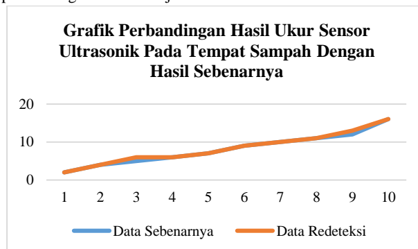
Gambar 13 Grafik Perbandingan Hasil Ukur Jarak Sampah dengan Ultrasonik dan Penggaris
