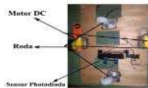
Gambar 10.b Hasil Rancangan Robot Pengumpul Sampah Otomatis Tampak Bawah
