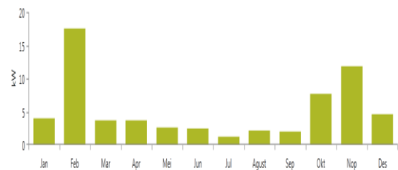
Gambar 1. Grafik Rata-Rata Daya Listrik yang dibangkitkan
