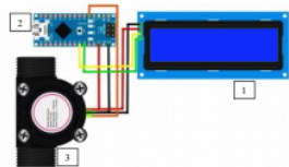
Gambar 3. Rangkaian Komponen Elektronik
