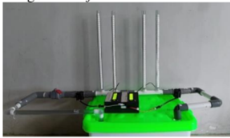
Gambar 4. Alat Peraga Asas Kontinuitas dengan Waterflow Sensor
