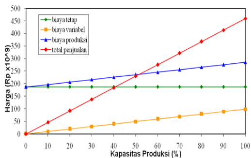
Gambar 5. Grafik Break Even Point Pabrik Pembuatan Biohidrogen
