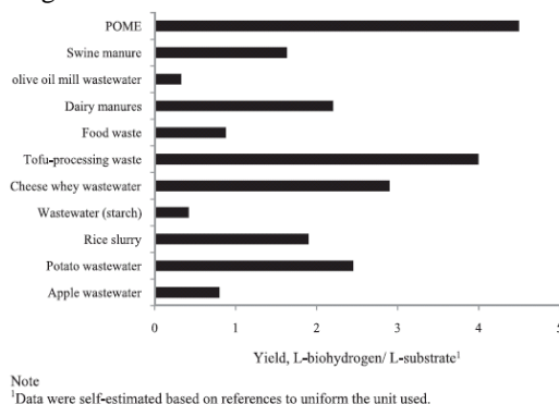
Gambar 1. Yield dari biohidrogen dengan menggunakan umpan yang berbeda [7]
