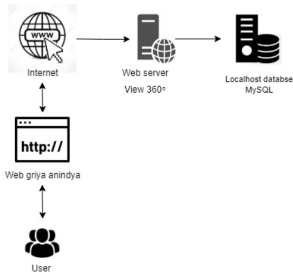
Gambar 2 Arsitektur Sistem
