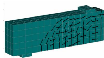
Gambar 16. Pola retak balok dengan sudut tulangan sengkang 120°
