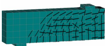
Gambar 12. Pola retak balok dengan sudut tulangan sengkang 60°
