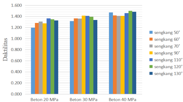
Gambar 10. Hasil nilai daktilitas balok beton bertulang
