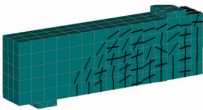
Gambar 17. Pola retak balok dengan sudut tulangan sengkang 130°
