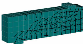
Gambar 11. Pola retak balok dengan sudut tulangan sengkang 50°
