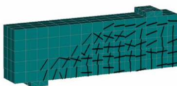
Gambar 13. Pola retak balok dengan sudut tulangan sengkang 70°
