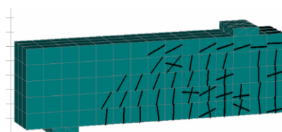
Gambar 15. Pola retak balok dengan sudut tulangan sengkang 110°
