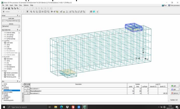
Gambar 6. Tampak balok setelah di FE Mesh
