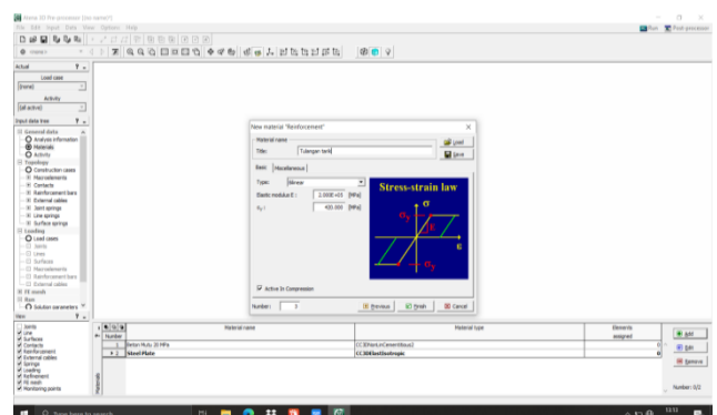
Gambar 3. Input material tulangan
