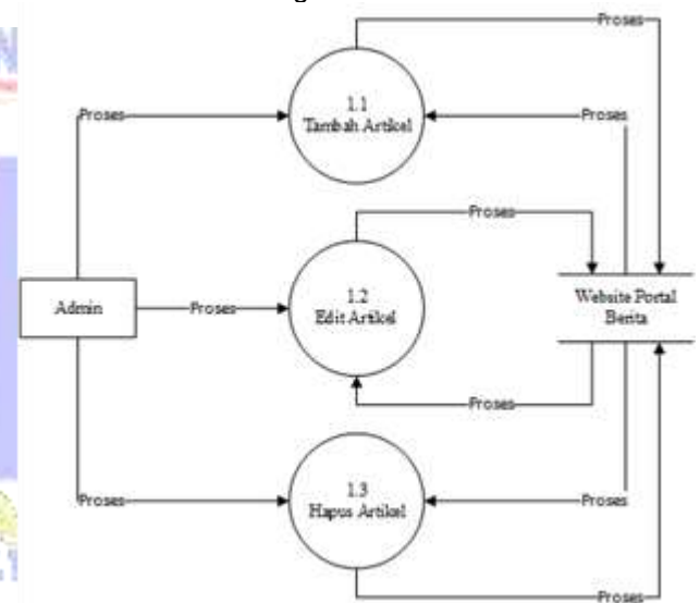
Gambar 4. DFD level 2
