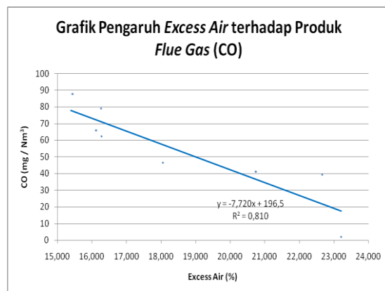
Gambar 7. Grafik Pengaruh Excess Air terhadap Produk Flue Gas ( CO )
