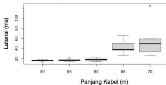
Gambar 5. Box plot latensi terhadap panjang kabel pada jaringan CAN tanpa pemancar-penerima.
