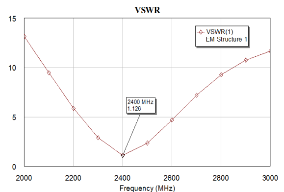
Gambar 4. Grafik simulasi VSWR antenna satu elemen peradiasi
