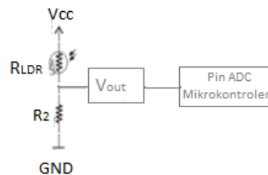
Gambar 3 Rangkaian sistem elektrik sensor LDR
