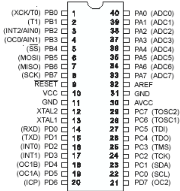
Gambar 7. Konfigurasi pin ATMEGA8535L Sumber: ATMEL,2006
