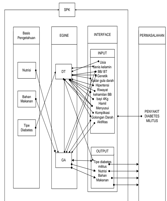
Gambar 2. Integrasi Decision Table dan Algoritma Genetika
