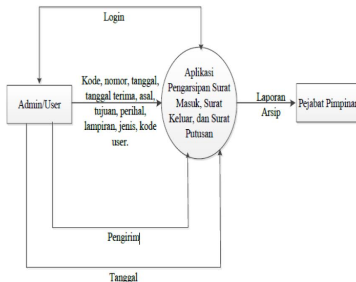
Gambar 1 Diagram Konteks
