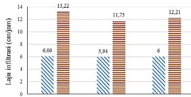
Gambar 6. Laju infiltrasi
