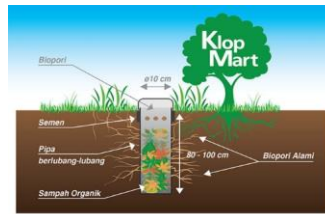
Gambar 5. Dimensi biopori pada umumnya
