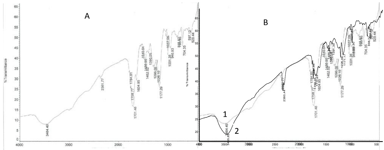
Gambar 2. A. Spektra IR PMAA; B(1). Spektra IR PMAA-BSA; B(2). Spektra IR imprinted PMAA-BSA
