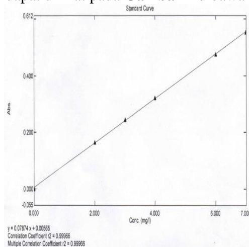
Gambar 2. Kurva Kalibrasi Larutan Kafein Baku dalam Aquadest
