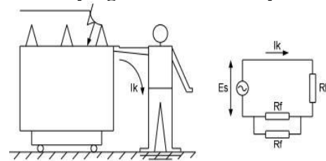
Gambar 4. Tegangan sentuh dan rangkaian ekuivalennya
