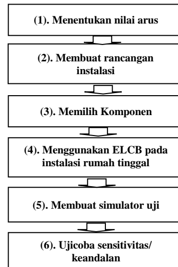
Gambar 10. Tahapan Rancangan ELCB
