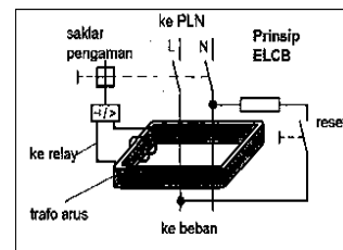
Gambar 3. Instalasi ELBC dalam rumah
