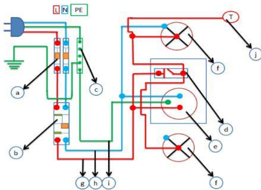
Gambar 11. Pengawatan Simulator
