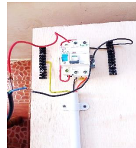
Gambar 12. Pemasangan ELCB pada instalasi
