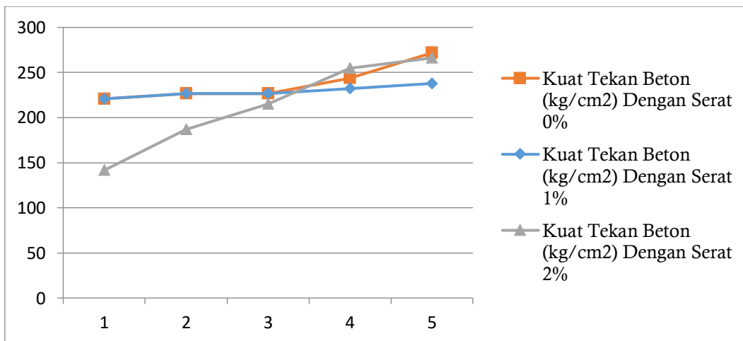
Gambar 5. Grafik Kuat Tekan Beton Dengan Serat 0%, 1% dan 2% Sumber : Peneliti, 2021
