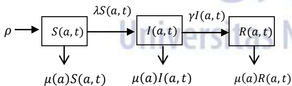
Diagram alur model epidemik SIR berdasarkan umur
