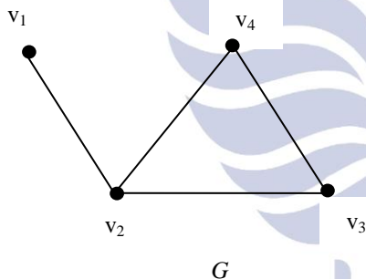
Gambar 3.1 Graf dengan empat titik dan empat sisi
