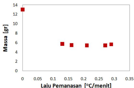
Gambar 4. Reduksi massa kotoran sapi dengan perbedaan laju pemanasan
