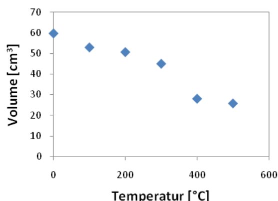
Gambar 7. Reduksi volume kotoran sapi pada perbedaan temperatur pirolisis
