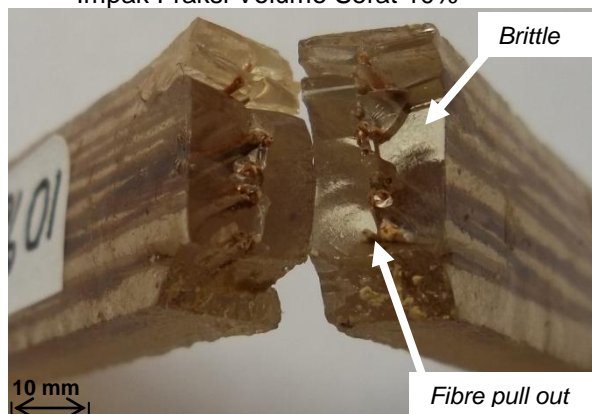
Gambar 16. Penampang Melintang Komposit Impak Fraksi Volume Serat 10%.
