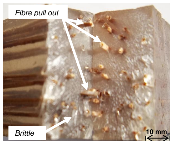
Gambar 10. Penampang Melintang Komposit Tarik Fraksi Volume Serat 10%.
