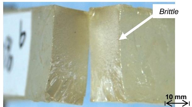
Gambar 8. Penampang Melintang Komposit Tarik Fraksi Volume Serat 0%.
