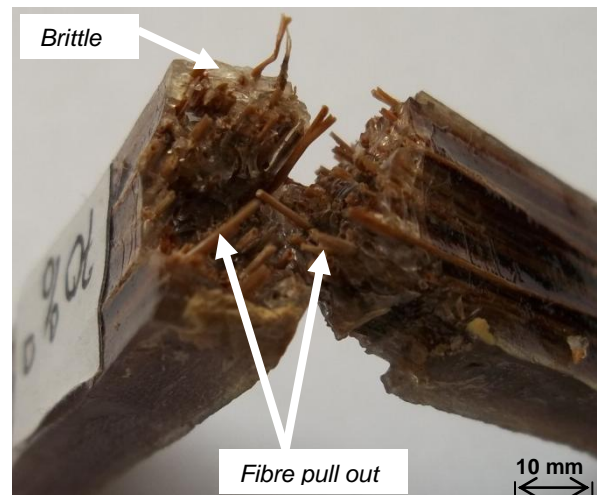
Gambar 18. Penampang Melintang Komposit Impak Fraksi Volume Serat 70%.
