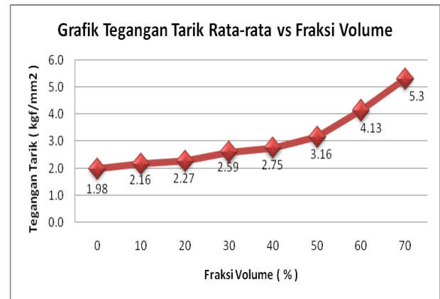
Gambar 2. Grafik Hubungan Tegangan Tarik rata-rata dan Fraksi Volume Serat
