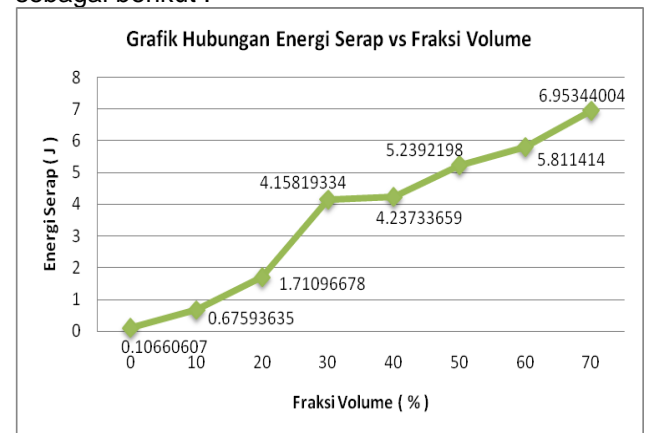
Gambar 5. Grafik Hubungan Energi Serap Rata-rata dan Fraksi Volume Serat
