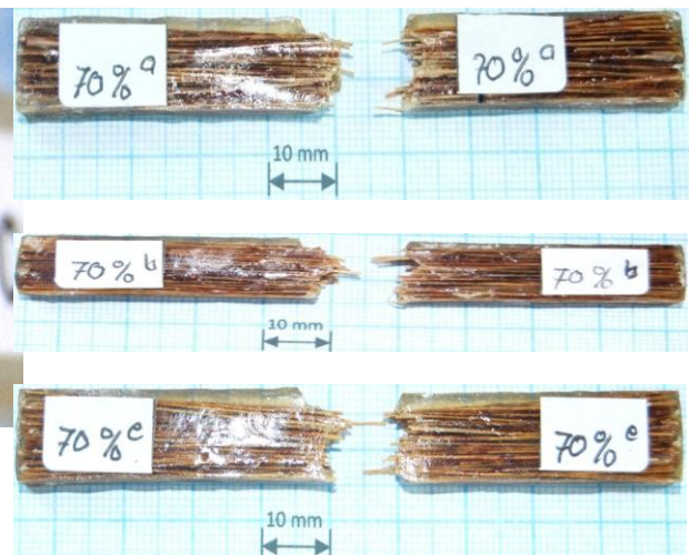
Gambar 17. Permukaan Patahan Komposit Impak Fraksi Volume Serat 70%
