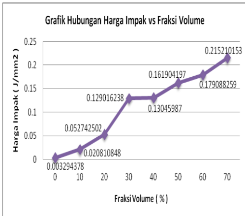
Gambar 6. Grafik Hubungan Harga Impak Rata-rata dan Fraksi Volume Serat
