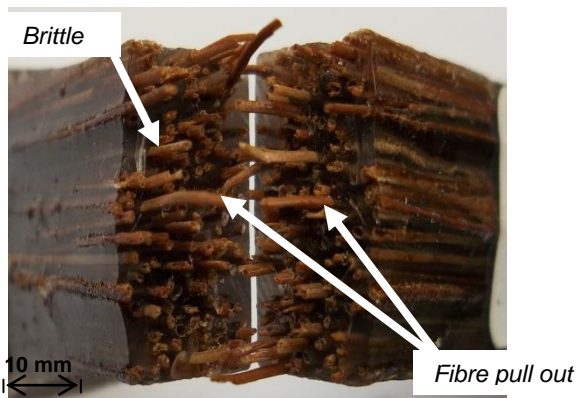
Gambar 12. Penampang Melintang Komposit Tarik Fraksi Volume Serat 70%.
