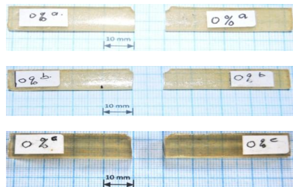
Gambar 13. Permukaan Patahan Komposit Impak Fraksi Volume Serat 0%
