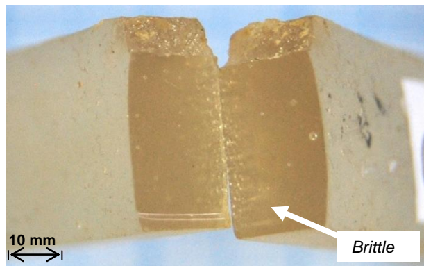
Gambar 14. Penampang Melintang Komposit Impak Fraksi Volume Serat 0%.
