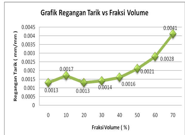
Gambar 3. Grafik Hubungan Regangan Tarik dan Fraksi Volume Serat
