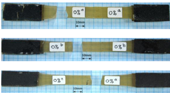
Gambar 7. Permukaan Patahan Komposit Tarik Fraksi Volume Serat 0%
