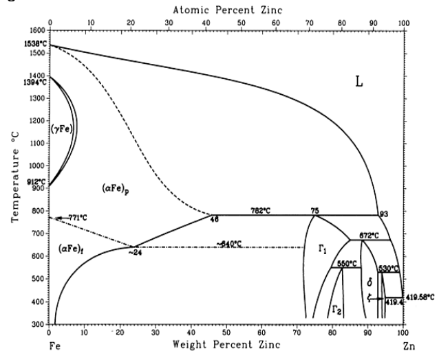
Gambar 1. Diagram Kesetimbangan Fe-Zn[3].
