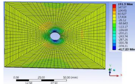
Gambar 2. Contoh distribusi tegangan sisa pada sekitar lubang dengan t = 1 mm dan D_p = 8.4 mm.
