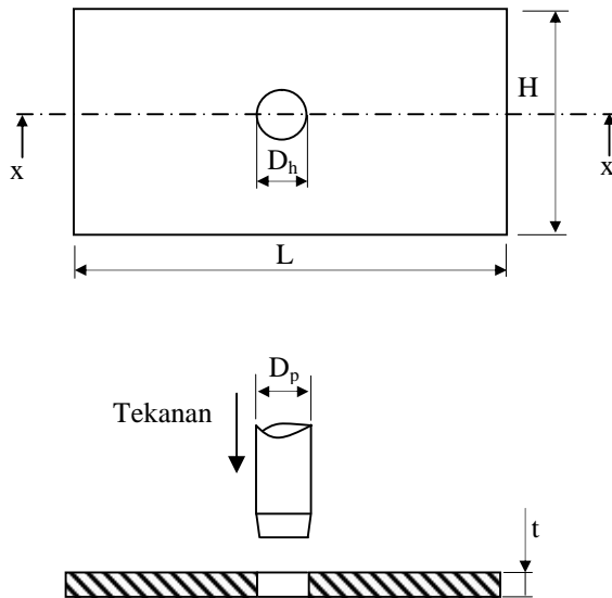
Potongan x-x
