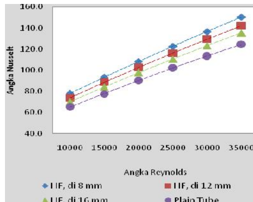
Gambar 6 – Grafik Pengaruh Diameter Inner-Helical Fin dan Plain Tube terhadap Perolehan Angka Reynolds dengan Peningkatan Angka Nusselt
