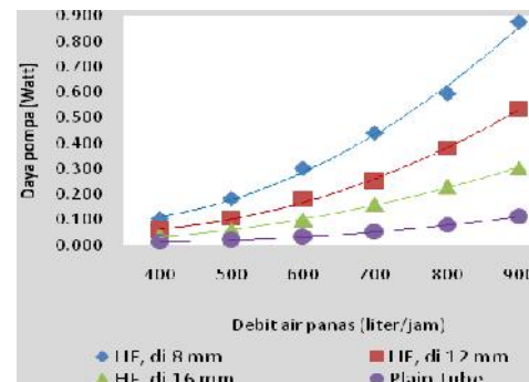
Gambar 4 – Grafik Pengaruh Diameter Inner-Helical Fin dan Plain Tube terhadap Daya Pompa (watt) di Tiap Debit Air Panas
