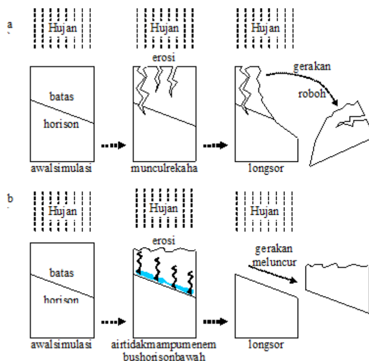
Gambar 6. Skema proses robohan (a) dan longsor (b)
