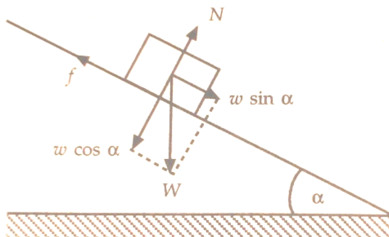
Gambar 2. Distribusi gaya pada kemiringan batas horison (Kamajaya, 1999)
