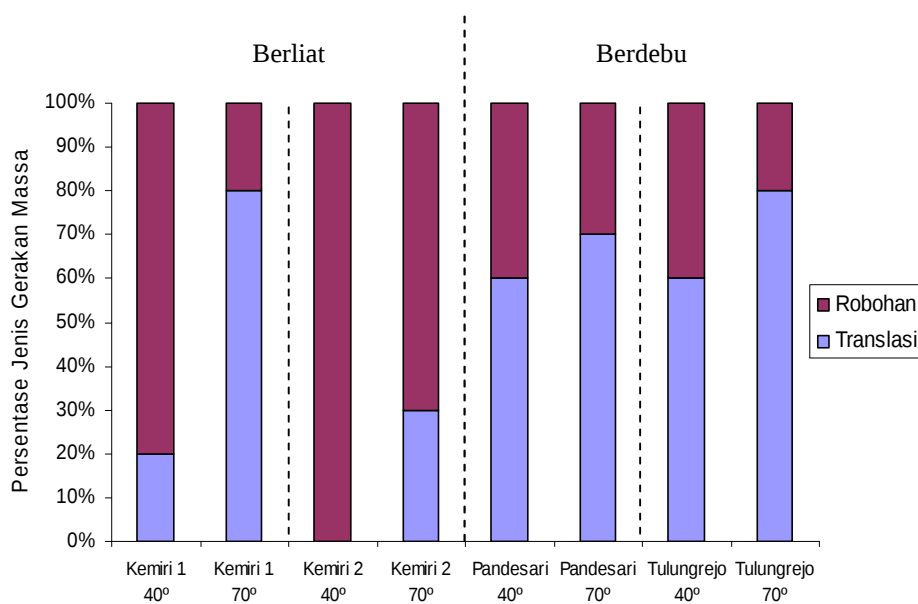
Gambar 5. Jenis gerakan massa yang terjadi pada saat simulasi longsor
