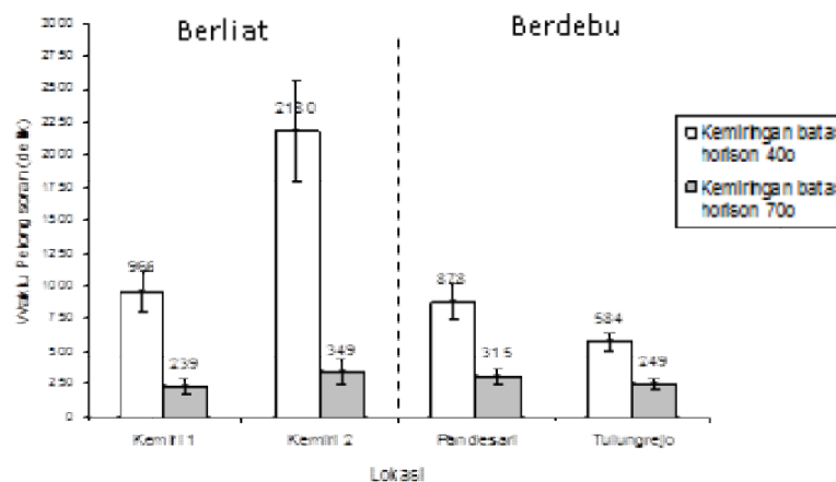
Gambar 1. Waktu pelongsoran rata-rata pada tiap lokasi dengan kemiringan batas horison 40° dan 70°
