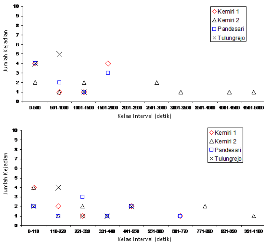
Gambar 4. Sebaran Waktu Pelongsoran pada Kemiringan Batas Horison 40° (atas) dan 70° (bawah)
