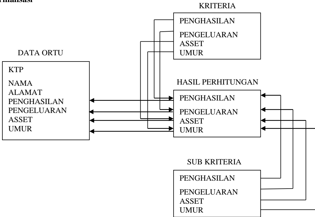
Gambar 3 Normalisasi Tahap 3
