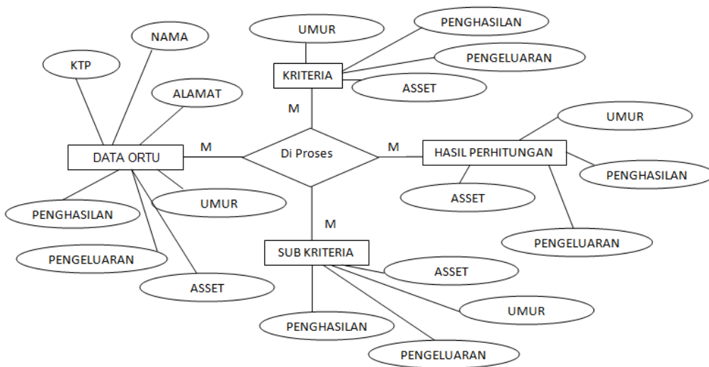
Gambar 4 ERD
