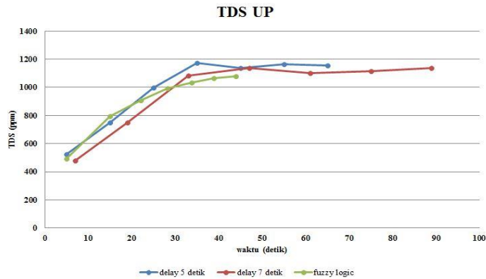
Gambar 12. Pengujian Menaikkan Kandungan TDS
