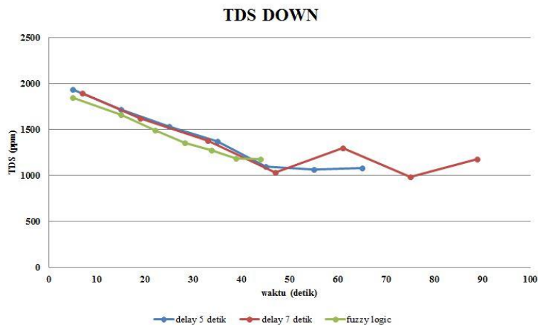
Gambar 13. Pengujian Menurunkan Kandungan TDS
