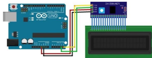
Gambar 4. Bagian Monitoring
