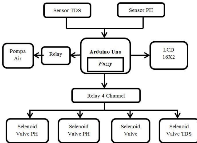
Gambar 1. Diagram Blok Sistem Keseluruhan
