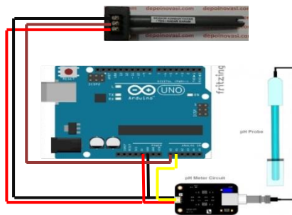
Gambar 2. Hubungn Sensor dengan Kendali Mikro
