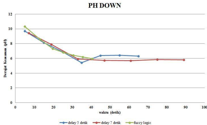
Gambar 11. Pengujian Menurunkan PH
