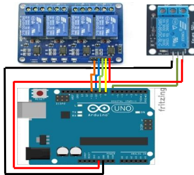
Gambar 3. Bagian Aktuator
