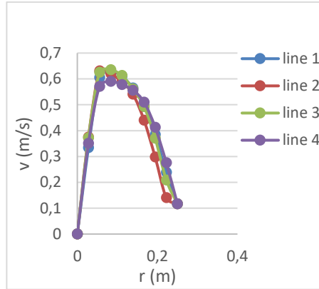
Gambar 10. Grafik Distribusi Kecepatan Pada Lubang Buang 2
