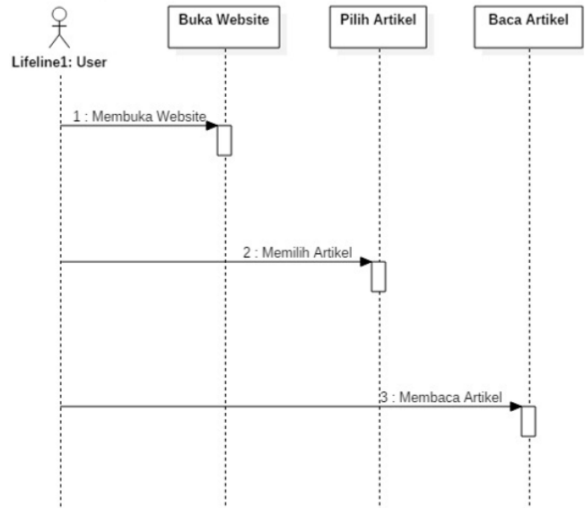
Gambar 4 Sequence Diagram Pengguna (User)
