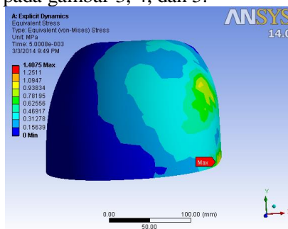
Gambar 3. Distribusi tegangan pada sisi depan helmet sepeda
