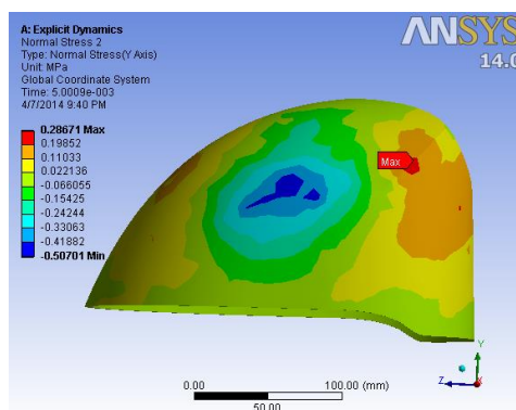
Gambar 8. Distribusi tengeran normal pada sumbu-y
