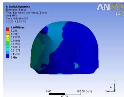
Gambar 5. Distribusi tegangan pada sisi belakang helmet sepeda
