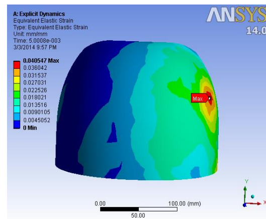
Gambar 23. Distribusi regangan pada sisi depan helm
