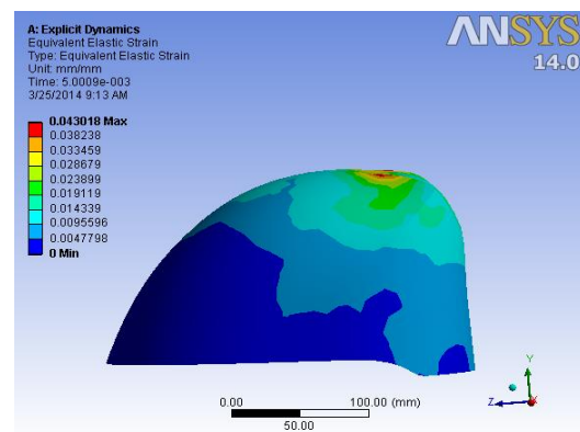
Gambar 24. Distribusi regangan pada sisi samping helm
