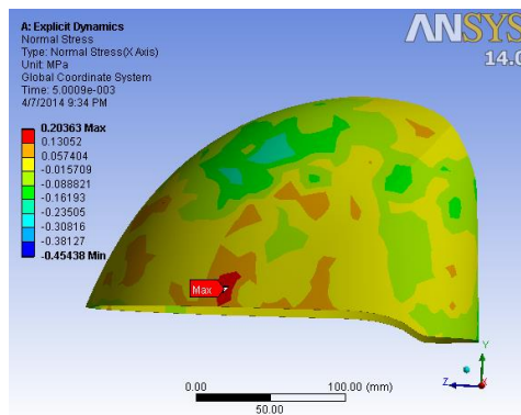
Gambar 7. Distribusi tengeran normal pada sumbu-x
