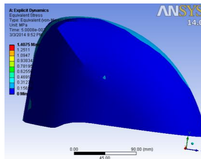
Gambar 4. Distribusi tegangan pada sisi kanan helmet sepeda
