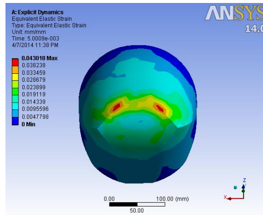
Gambar 22. Distribusi regangan pada sisi belakang helm sepeda
