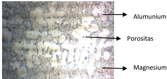
Gambar 4.16 Struktur mikro Al-Mg pada pembesaran 200X dengan tekanan O 2 11lb,c2h 2 3lb/m 2
