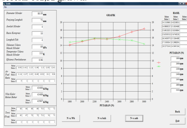
Gambar 3.7 Grafik Putaran vs Efisiensi Termal
