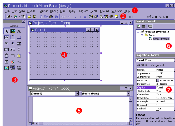
Gambar 2.2. IDE VB 6
