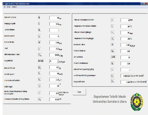
Gambar 3.2 Tampilan input
