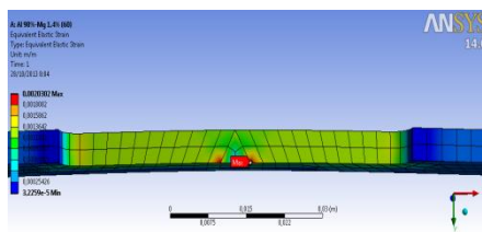
Gambar 10 Simulasi regangan
