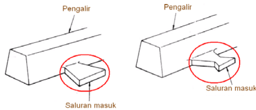
Gambar 2. Saluran masuk
