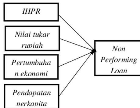
Gambar 1 Kerangka Berpikir
