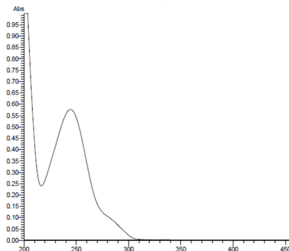
Gambar 2. Spektrum UV Panadol ®
