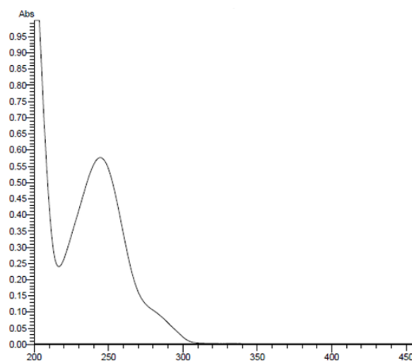
Gambar 1. Spektrum UV Parasetamol BPF1
