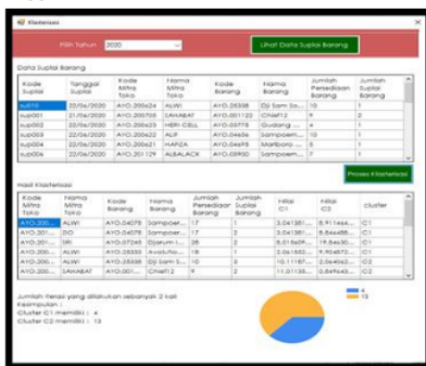
Gambar 8. Klasterisasi
